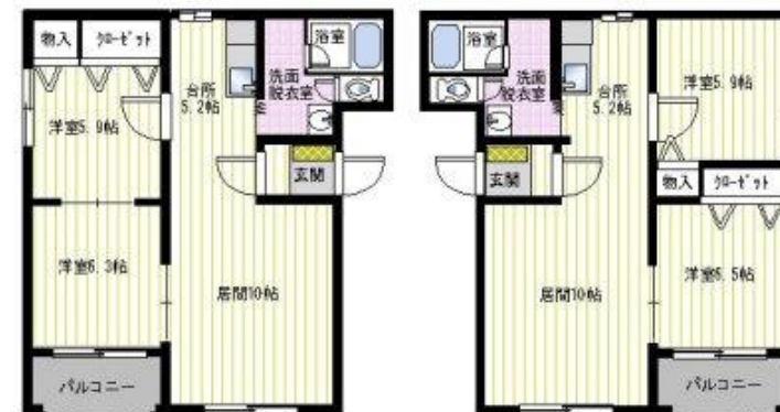
1号室タイプ
